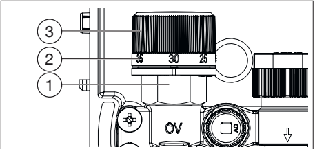
Fig. 4: Poignée manuelle
