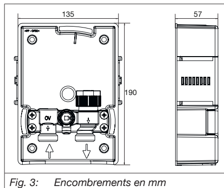
Fig. 3: Encombrements en mm
