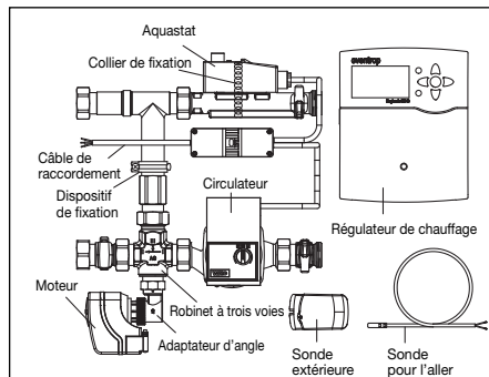
Fig. 5.1 Vue d'ensemble «Regufloor HW»
