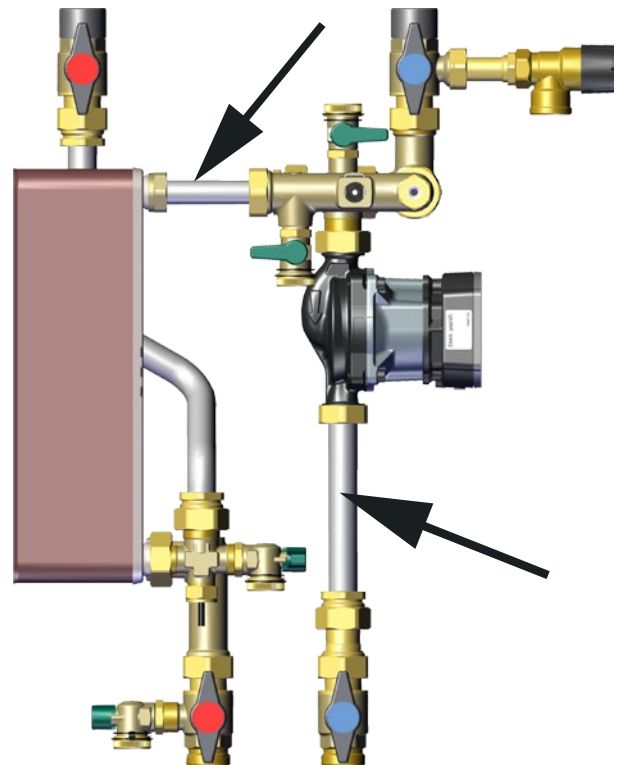
Fig. 17: Conexión equipotencial
