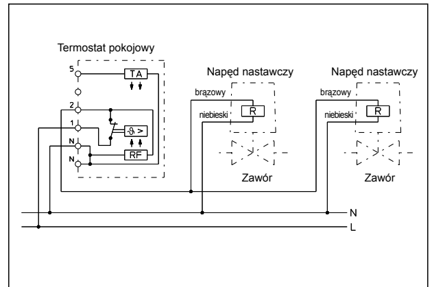
Schemat podłączenia
