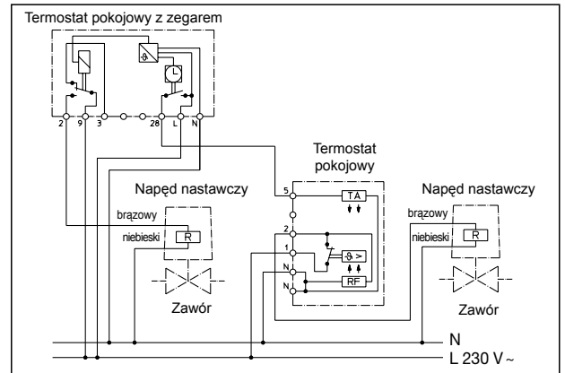
Schemat podłączenia
