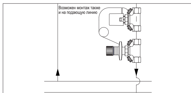
Пример: Регулирование расхода с помощью регулятора перепада давления „Нусосон DP“ и регулирующего вентиля „Нусосон TM“.
