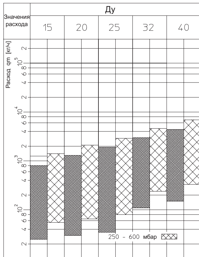
„Hydromat DP“ (50–300 мбар)/„Hycocor V“ „Hydromat DP“ (250–600 мбар)/„Hycocor V“
