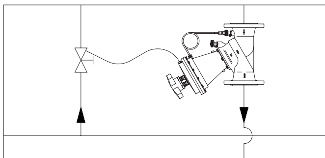
Пример: Регулирование перепада давления в системе с применением арматуры фланцевого типа.
