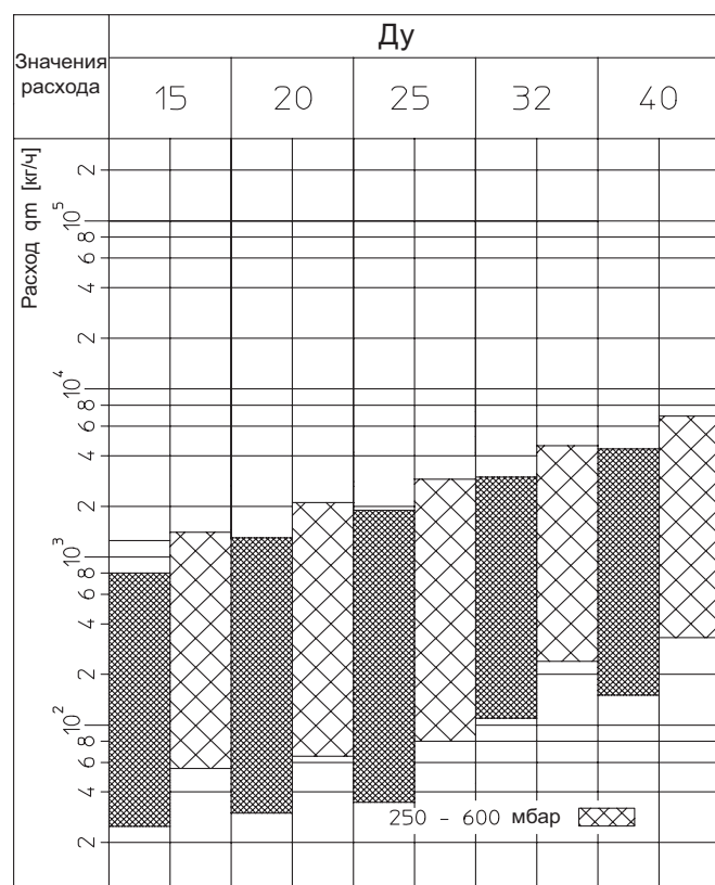
„Нусосон DP“/„Нусосон V“
