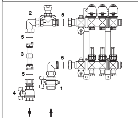
Illust. 3: Jeu de raccordement no. 1 pour compteurs de calories, modèle équerre, fournitures et placement des composants pour raccordement à droite
