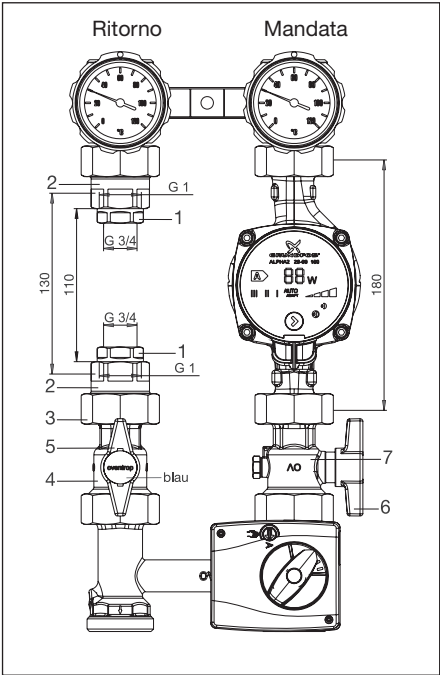
Fig. 5.2 Set installazione contacalorie per “Regumat M3-180” DN25 con valvola a sfera prima della pompa (2015)
