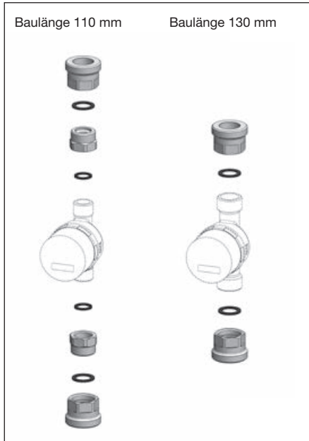
Abb. 5.3 Montage Wärmemengenzähler-Einbauset
