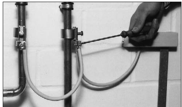
Bild 9: Für Potentialausgleich Erdungsschellen an beiden Solarkreisrohren anbringen und mind. 6 mm² Kabel mit Hauptpotentialausgleichsschiene verbinden.
