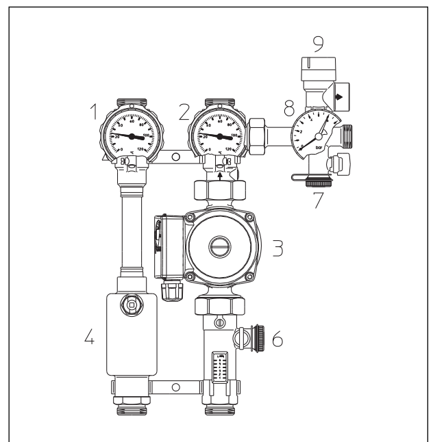
Bild 23: „Regusol L“-Solarstation
