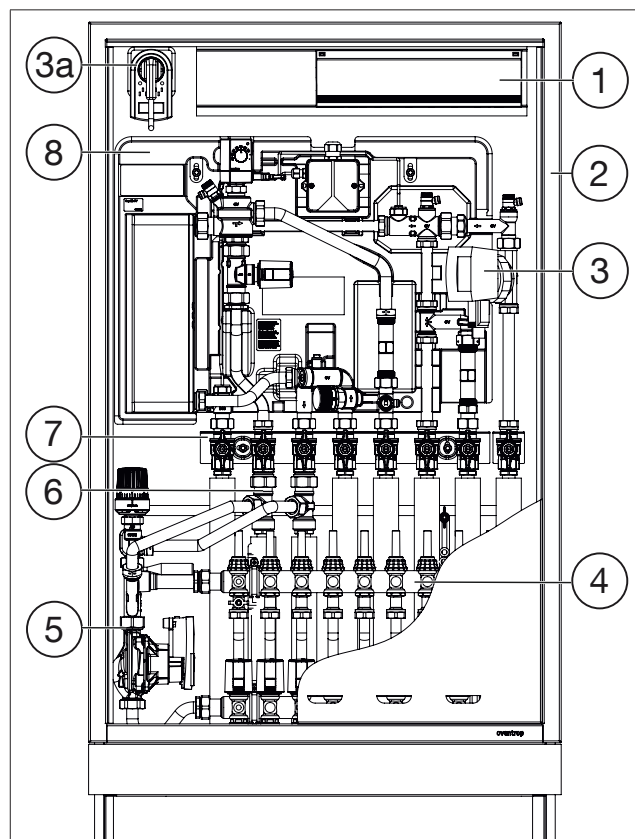
Abb. 3: Systembeispiel
