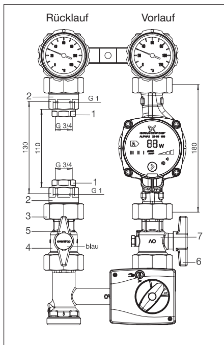
Abb. 5.2 Wärmemengenzähler Einbau – Set für „Regumat M3-180“ DN 25 mit Pumpenkugelhahn (2015)
