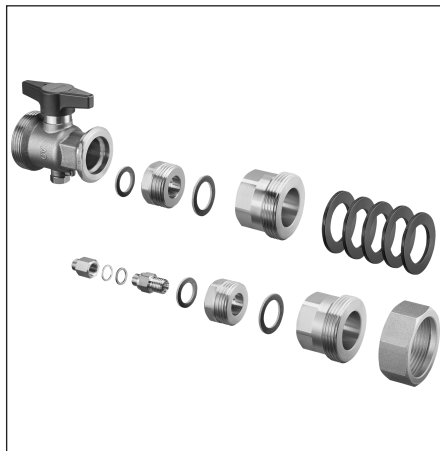
Fig. 1.1 Jeu de montage pour compteurs de calories DN 25 (2015)
