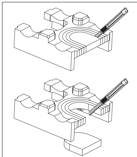
Fig. 5.4 Bloc d'insertion avec découpe pour compteur de calories
