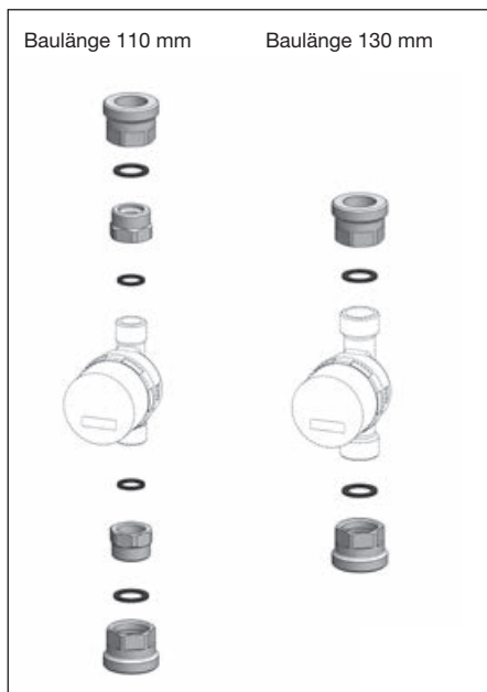
Abb. 5.3 Montage Wärmemengenzähler-Einbauset
