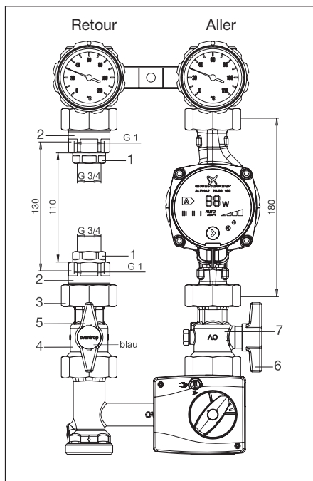
Fig. 5.2 Jeu de montage pour compteurs de calories pour «Regumat M3-180» DN 25 avec robinet d'isolement à tournant sphérique (2015)
