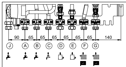
Abb. 4.4 Anschlussmaße
