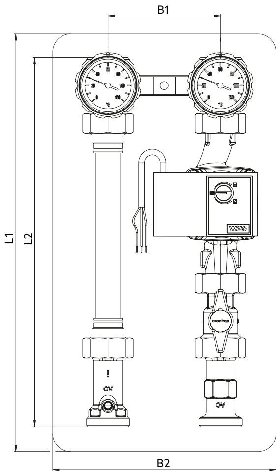
Fig. 5: Encombrements Regumat S
