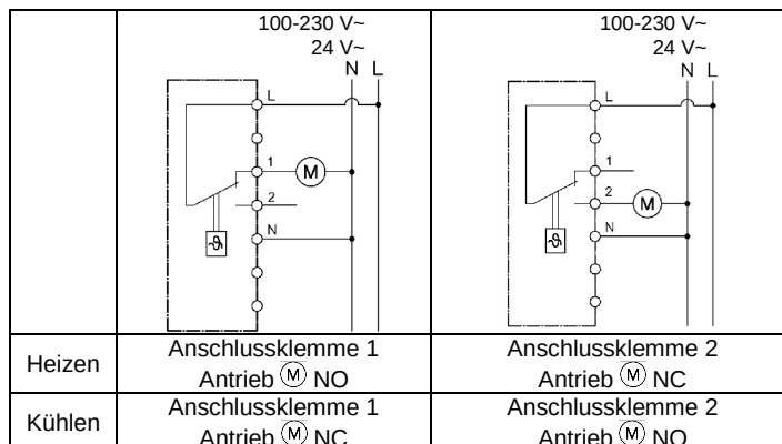
Abb. 6.2 Schaltplan Heizen/Kühlen
