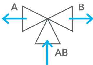
Toepassing als verdeelafsluiter: stroom AB wordt tussen A en B verdeeld, afhankelijk van de stand
