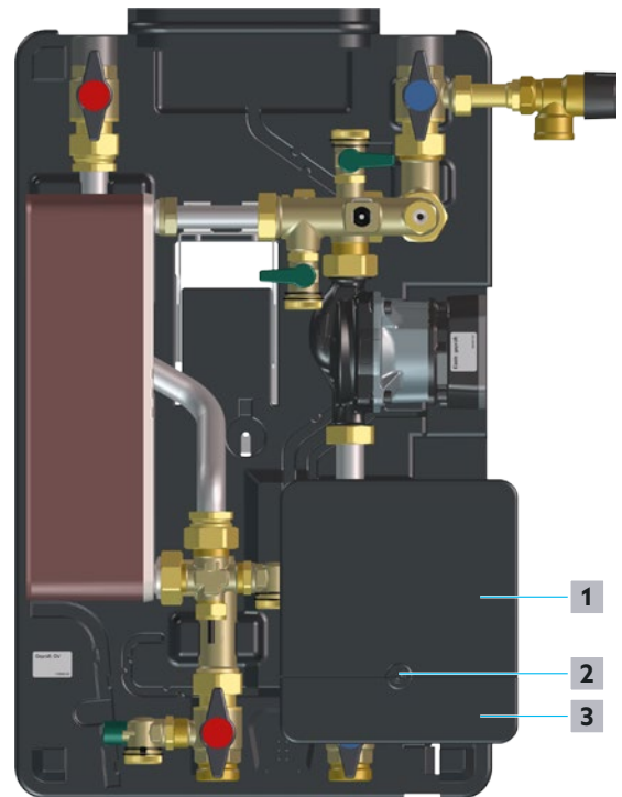
Fig. 22: Ouverture du régulateur
