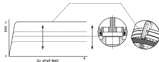
Fig. 4: Pression différentielle p_1-p_3 (bar)
