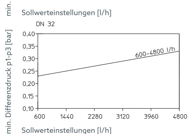
Abb. 13: Minstdifferenzdrücke
