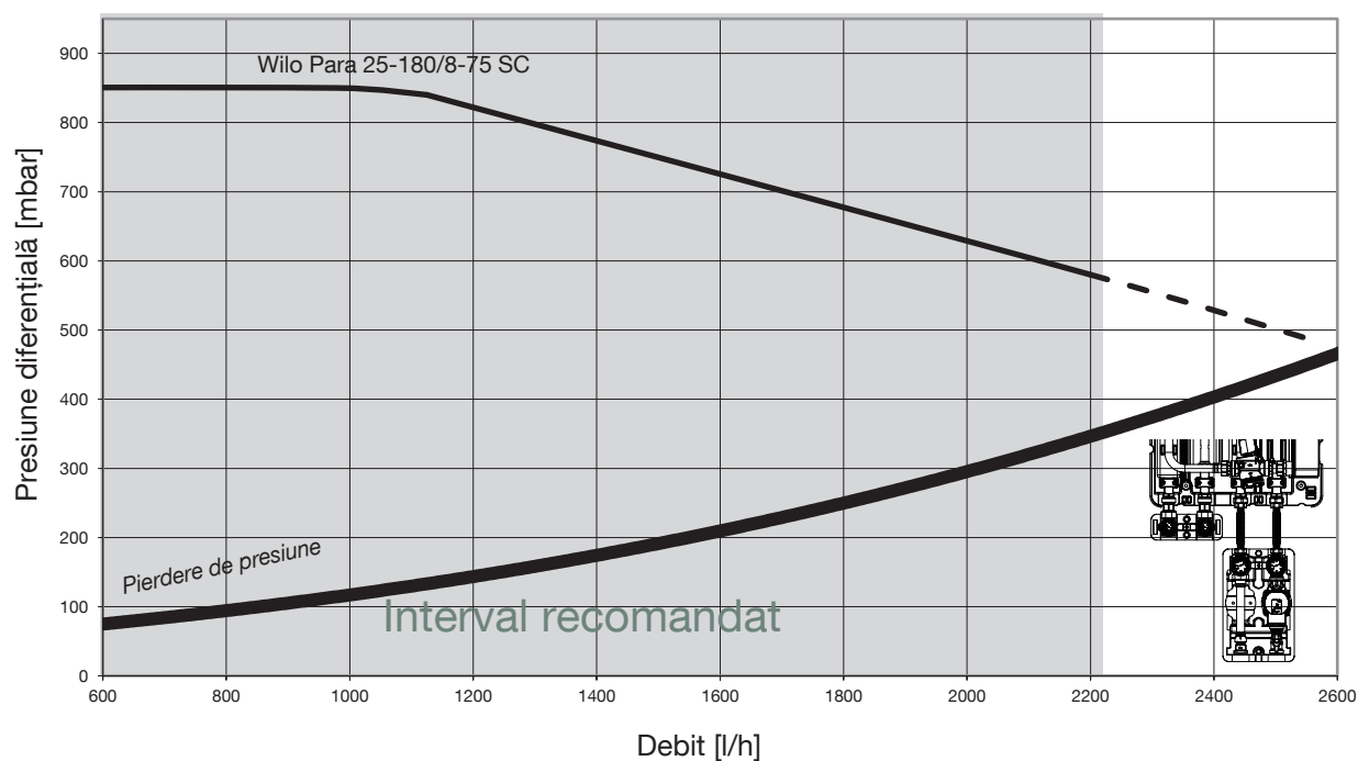
Fig. 5: Pierdere de presiune circuit secundar Regudis H-H
