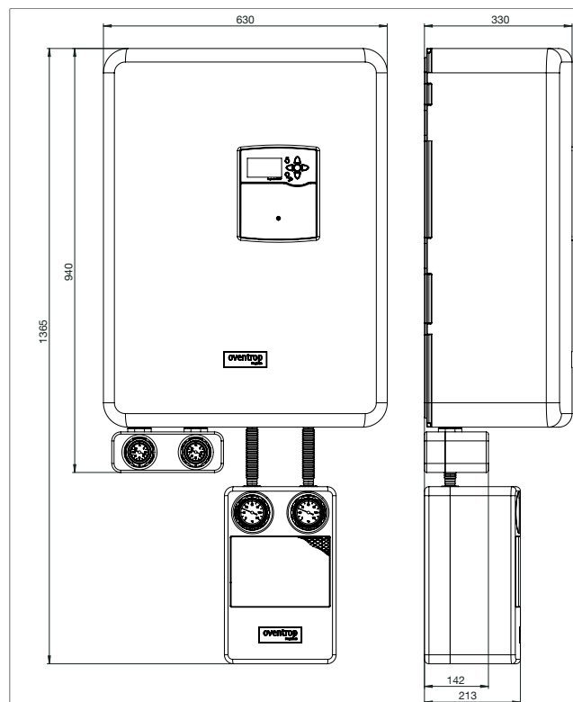
Fig. 3: Dimensiuni în mm
