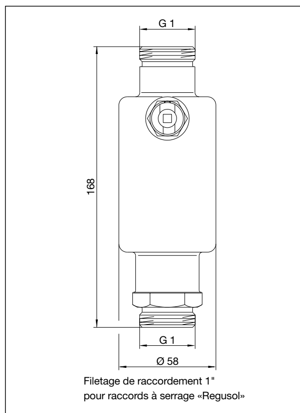
Pot de purge «Regusol»
