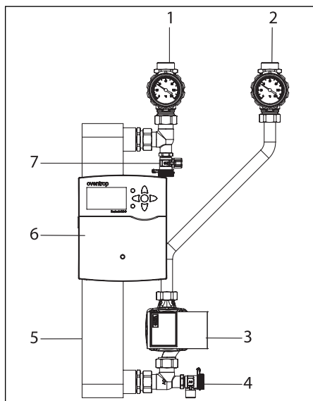
Fig. 17: Riempimento, svuotamento
