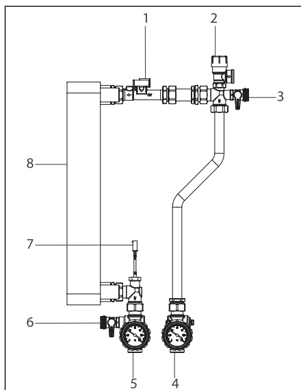
Fig. 18: "Regumaq X-30-B" riempimento e sfiato
