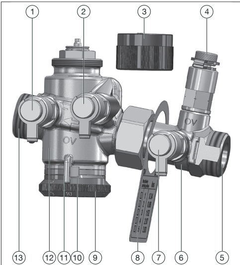
Abb. 1: « Cocon QTZ » avec diaphragme de mesure
