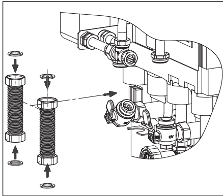
Abb. 14 Montage Metallwellrohre
