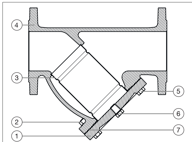
Abb. 1: Schmutzfänger Aufbau
