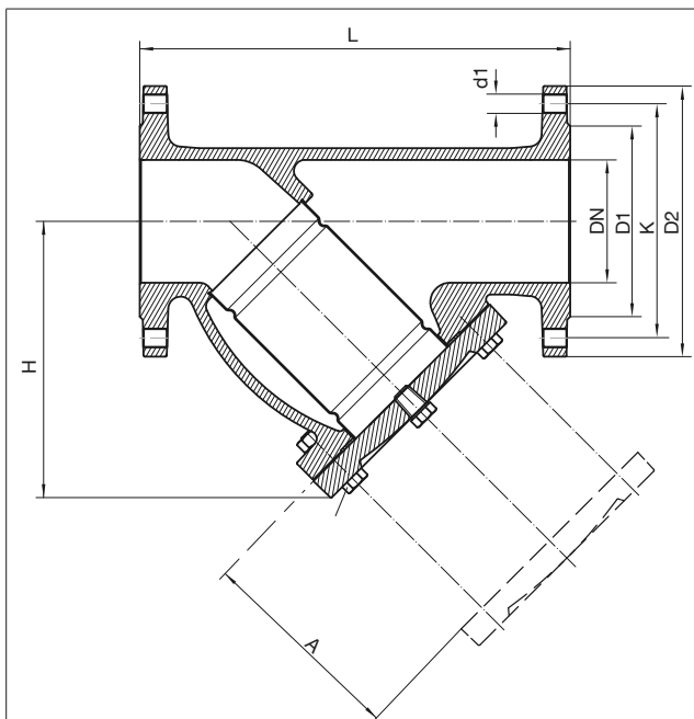
Abb. 2: Abmessungen
