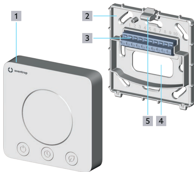
Abb. 3: Aufbau
