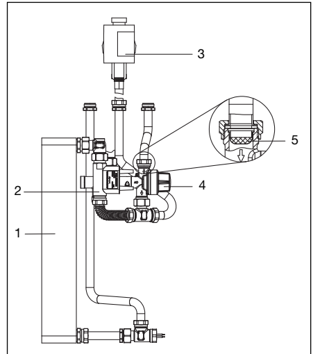
Abb. 5.3: Sekundärkreislauf
