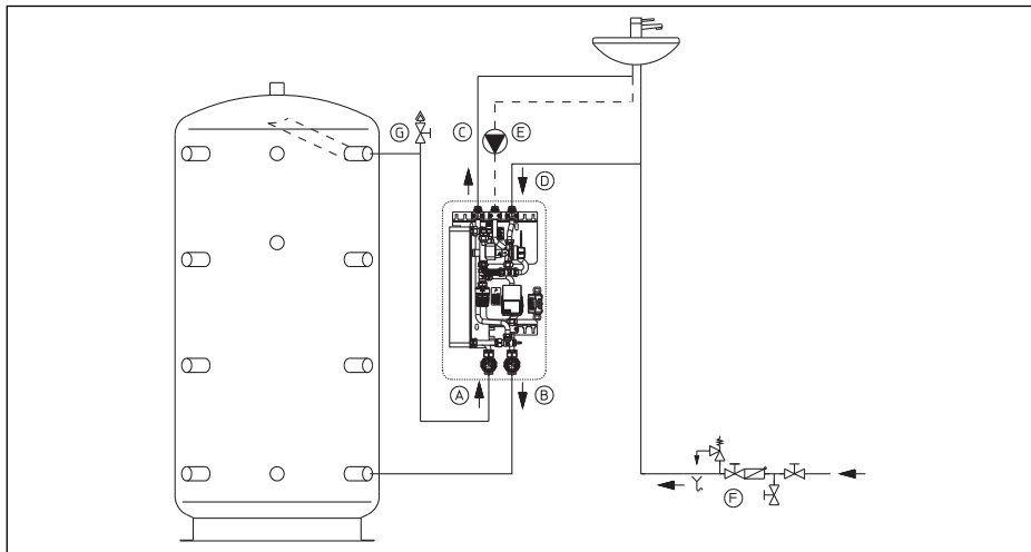
Abb. 5.6: Systemdarstellung
