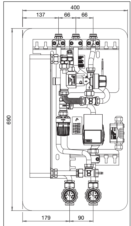
Abb. 6.1: Montage, Angaben in mm
