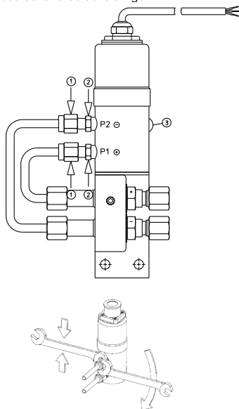
Abb. 5: Entlüftungsangabe
