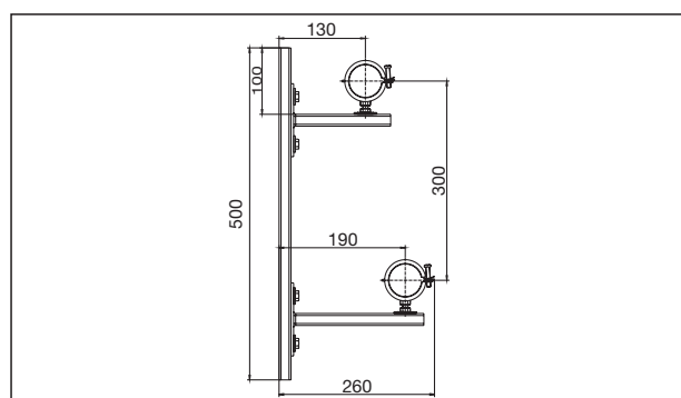
Maße Konsole
