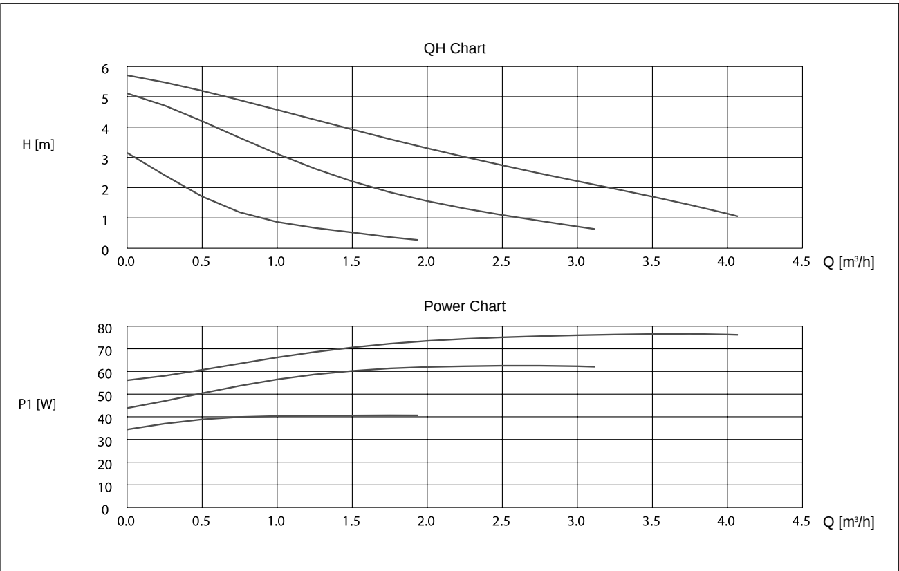
Grundfos Solar 15-60 130
