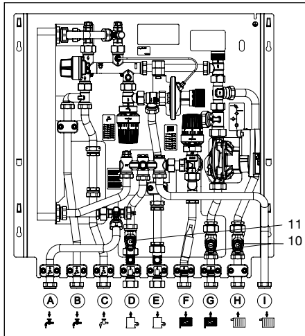
Abb. 8.1 Einbauposition Schmutzfänger
