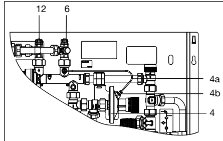
Abb. 8.2 Entlüftung
