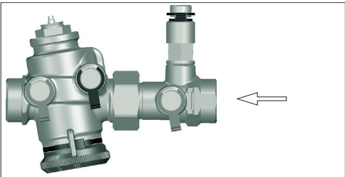
Abb. 13: Überwurfmutter anziehen
