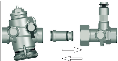
Abb. 12: Messblendeneinsatz wechseln
