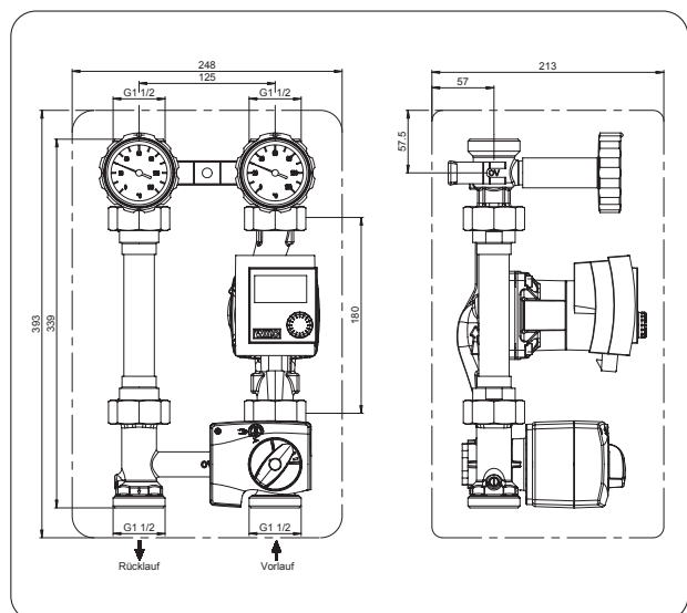
Regumat M3-180 DN 25 - modèle court
