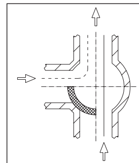
Principe de la fonction de mélange
