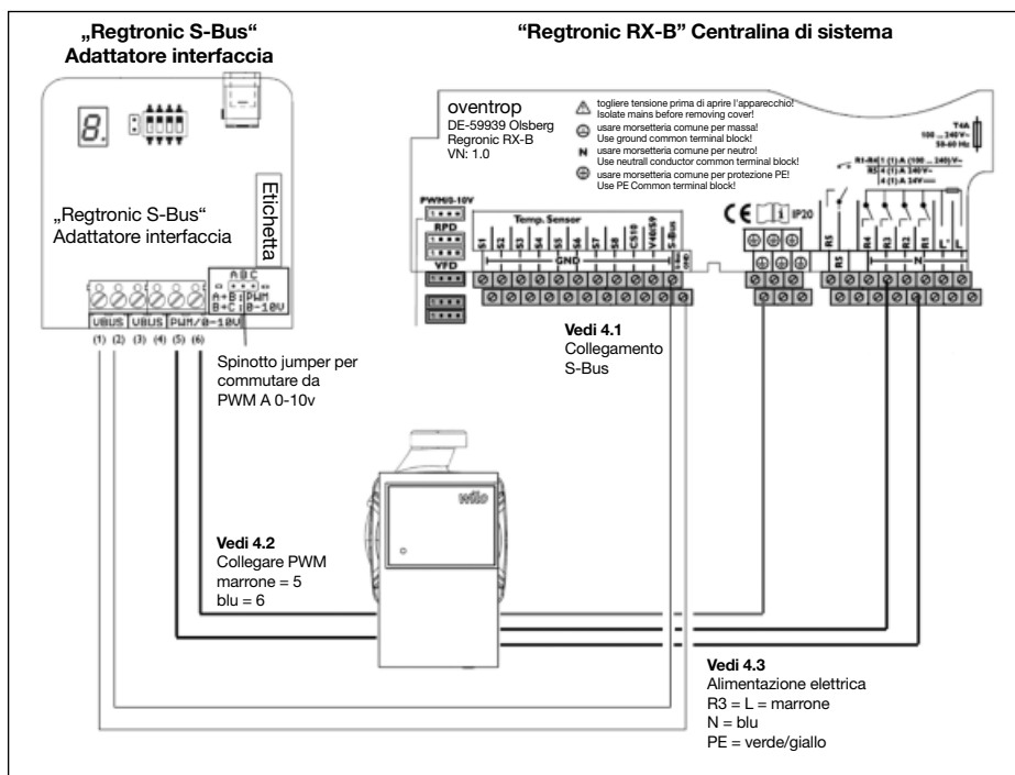
Fig. 5.4 Schema collegamento
