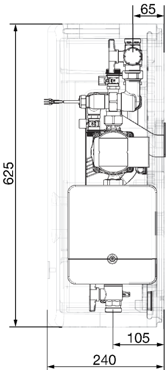
Dimensiuni Regumaq X-25 (vedere laterală)
