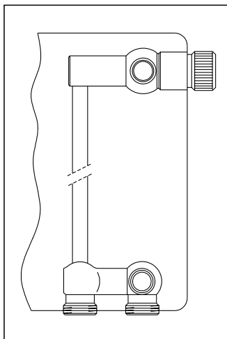
Grzejniki zaworowe z króćcami \frac{1}{4} ” GZ, rozstaw osi rur 50 mm
