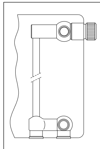
Grzejniki zaworowe z króćcami \frac{1}{2} ” GW, rozstaw osi rur 50 mm.
