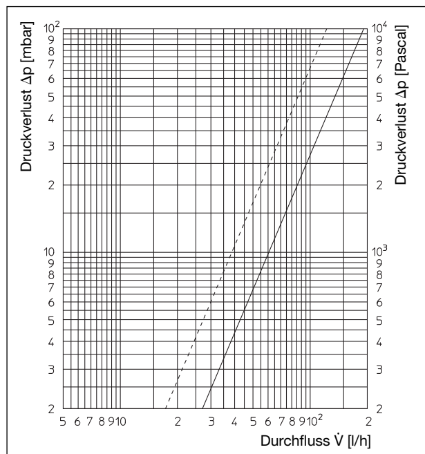
Durchflussdiagramm (Heizöl EL):
