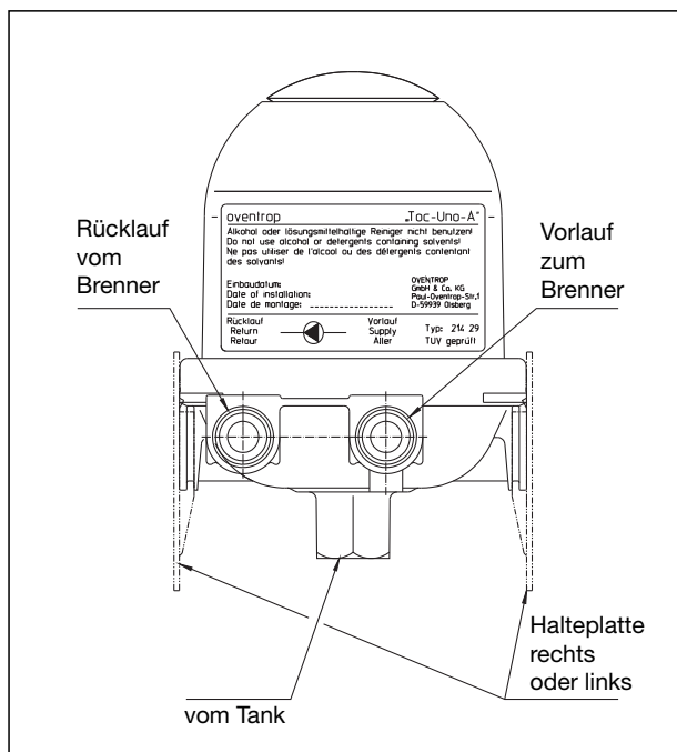
Ansicht Brennerseite
