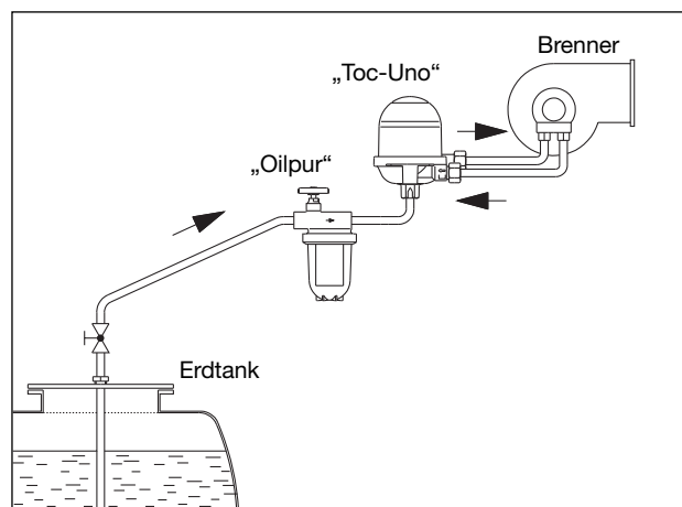
System-Darstellung: Installation des „Toc-Uno“ oberhalb des Ölspiegels
