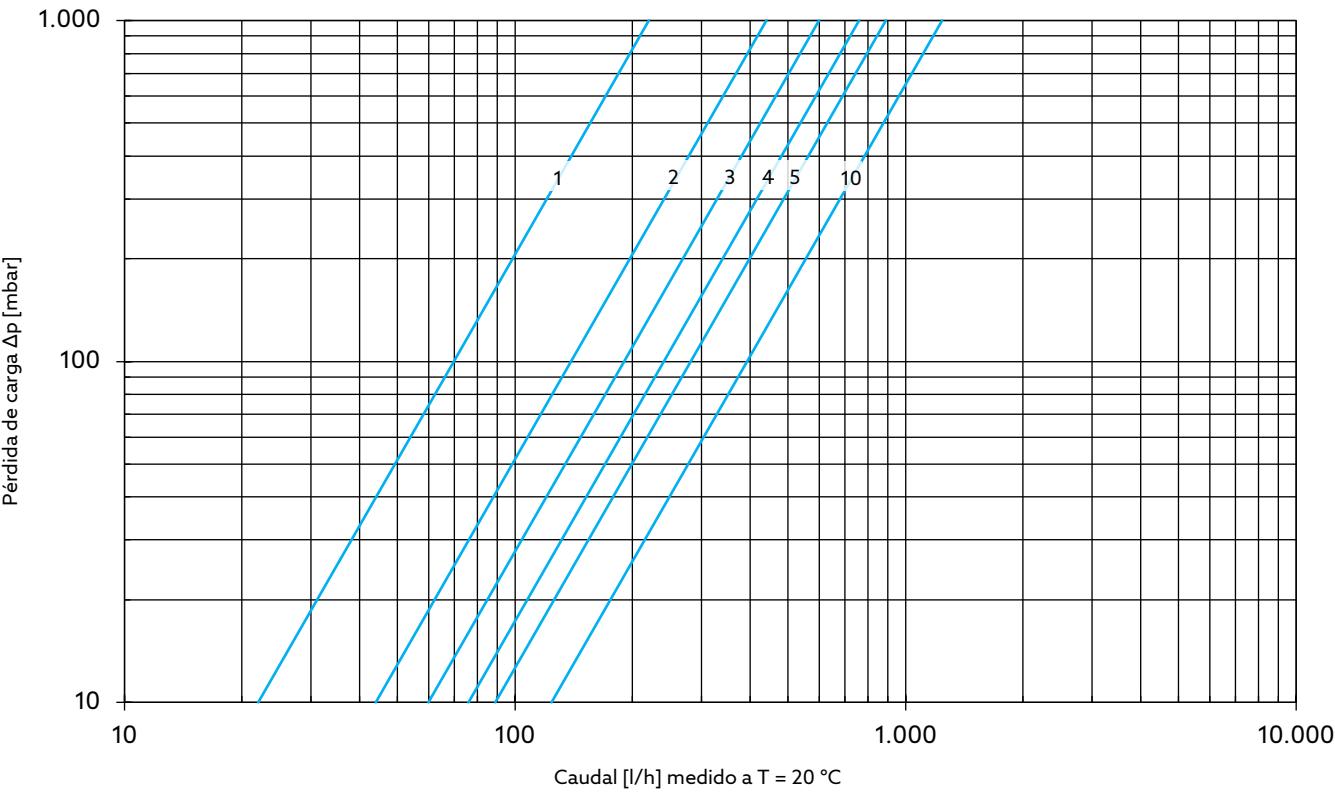
Valores de preajuste de caudal Aquastrom TV DN 15
