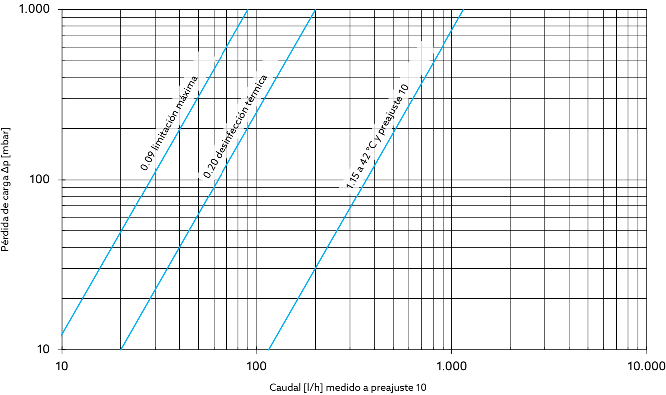
Control térmico del caudal Aquastrom TV DN 15
