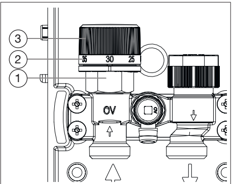
Fig. 4: Poignée manuelle
