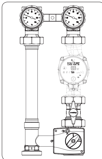
„Regumat M3-180“
