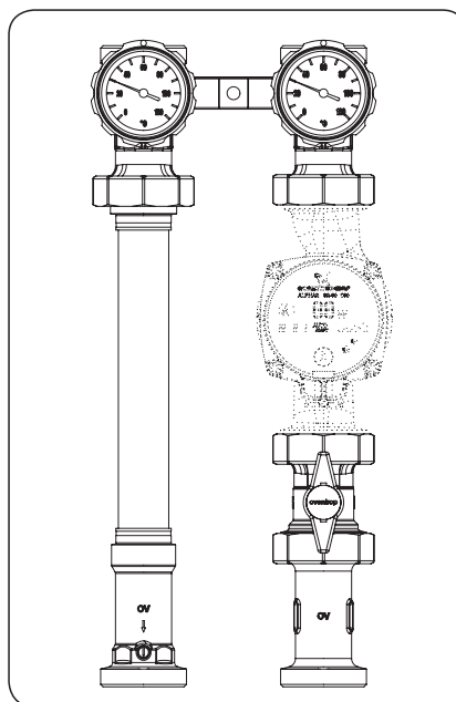
„Regumat S-180“
