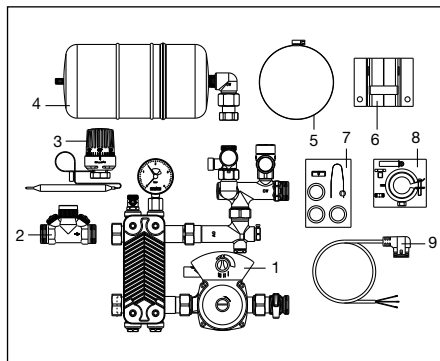
Abb. 5.1: Lieferumfang
