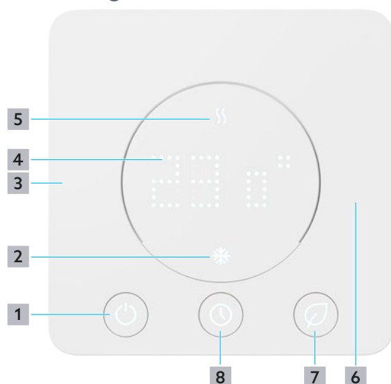
Fig. 4: Éléments de commande F 316
