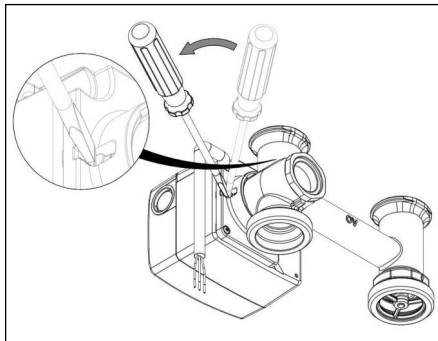
Abb. 5.3 Demontage Stellmotor
