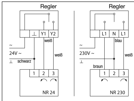
Abb. 5.1 Anschluss-Schema Dreipunktsteuerung
