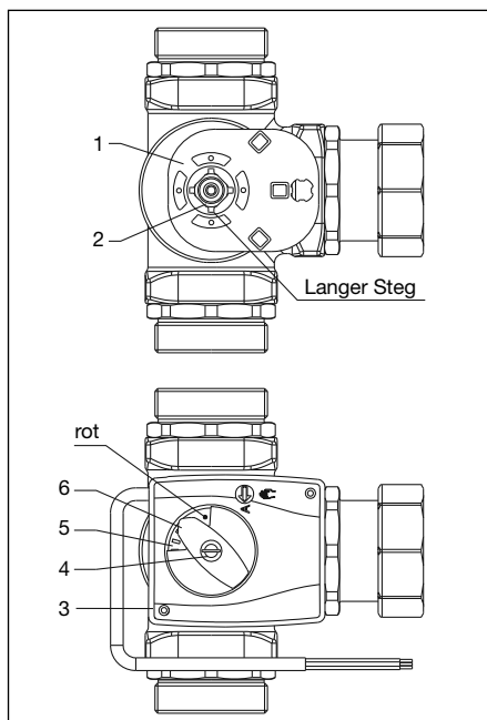
Abb. 5.8 Montage 3-Wege-Mischhahn DN40 / DN50
