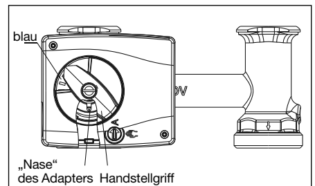
Abb. 5.5 3-Wege-Mischhahn Vorlauf links
