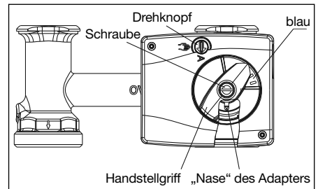
Abb. 5.4 3-Wege-Mischhahn Vorlauf rechts
