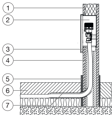
Fig. 5: Vue transversale de l'installation
