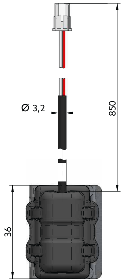
Fig. 2: Encombrements
