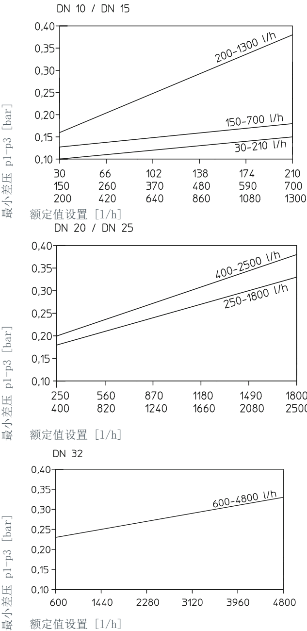
图 13: 最小差压
