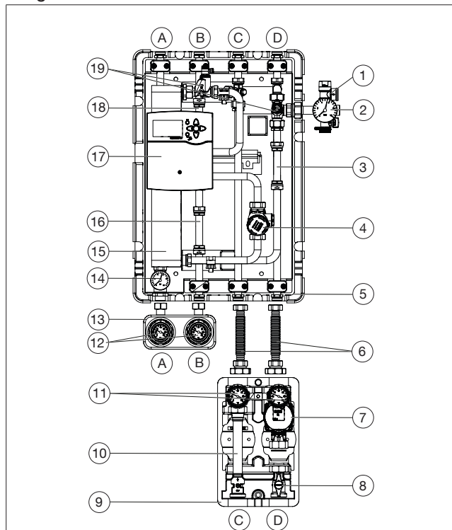
Abb. 2: Aufbau Regudis H-M
