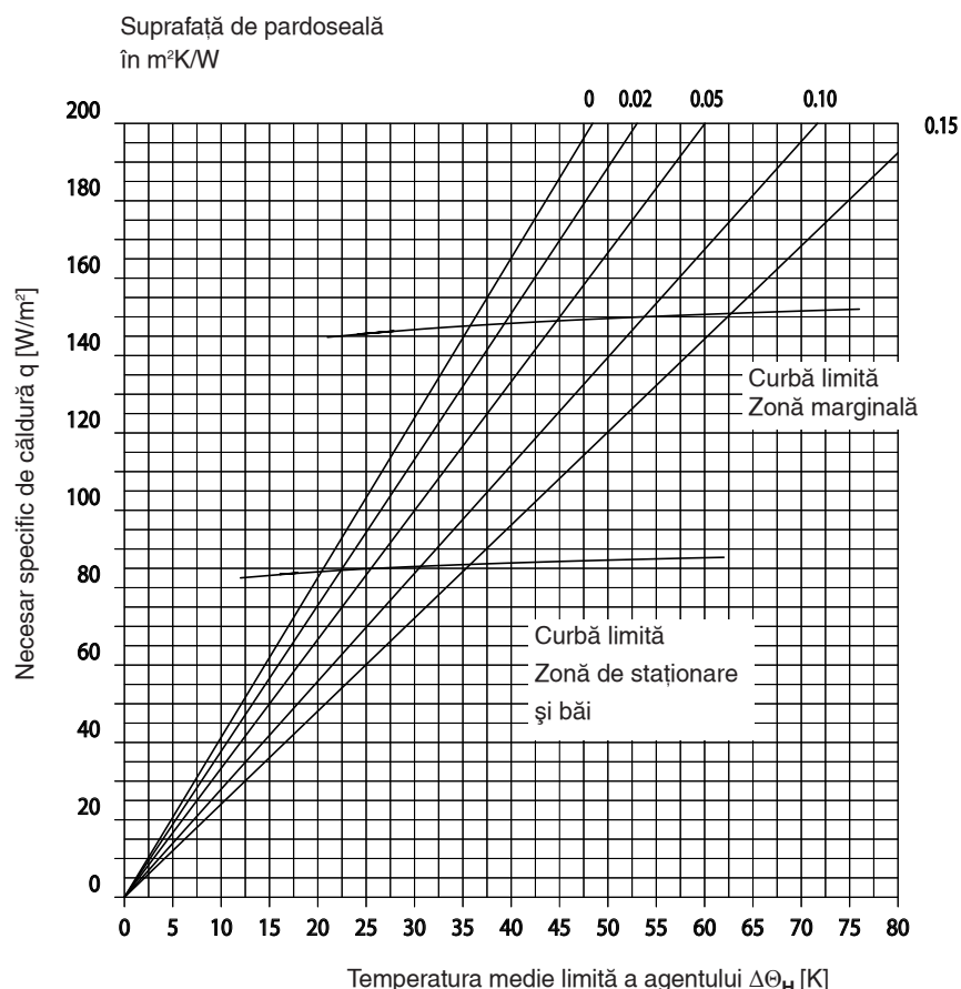
Diagrama de performanță pentru distanța de pozare a țevilor 125 mm
