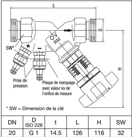
Fig. 4.1 Encombrements «Hydrocontrol STR» avec raccordement à serrage
