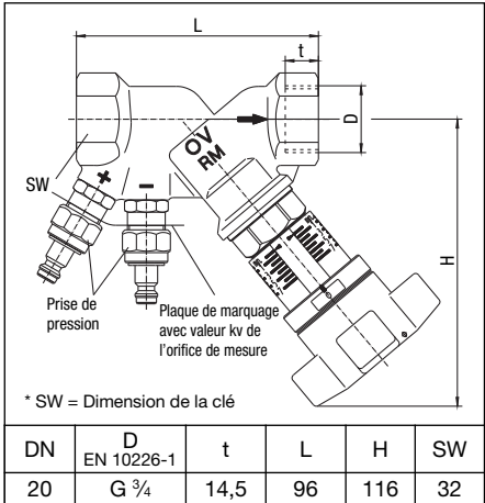
Fig. 4.2 Encombrements «Hydrocontrol STR» avec raccordement fileté femelle
