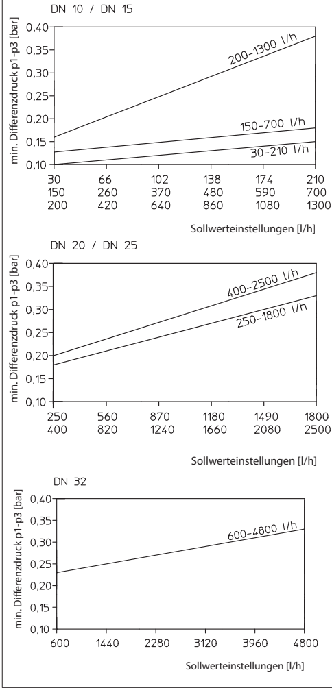
Abb. 13: Mindest-Differenzdrücke
