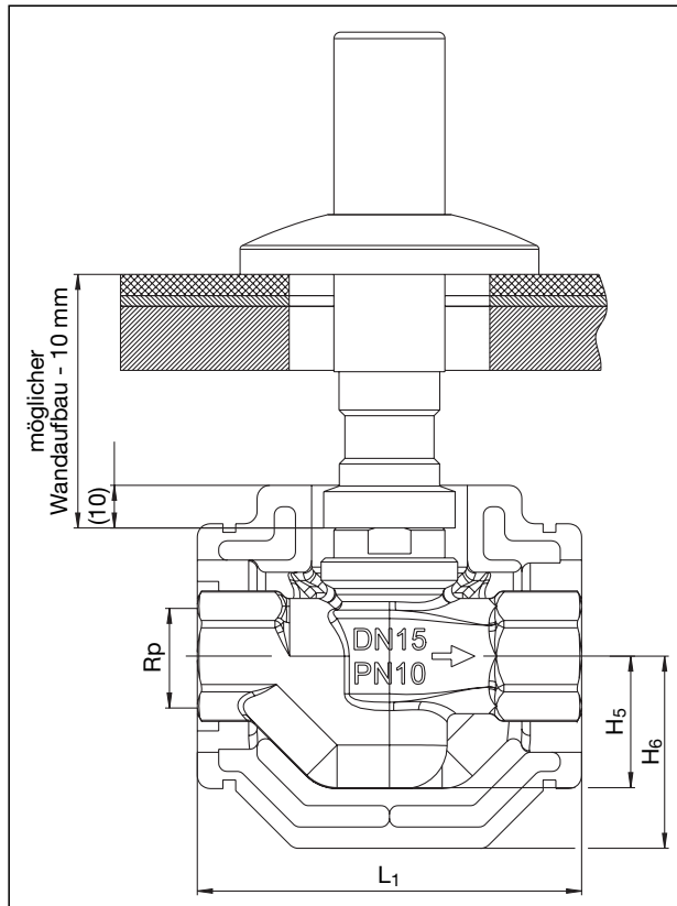
Maße „Aquaström UP-F“ mit Behördenoberteil fehlende Maße siehe Tabelle Seite vor
