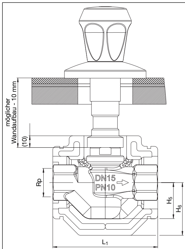
Maße „Aquaström UP-F“ mit Griffoberteil fehlende Maße siehe Tabelle Seite vor
