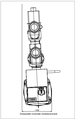
Einbautiefe innerhalb Verteilerschrank
